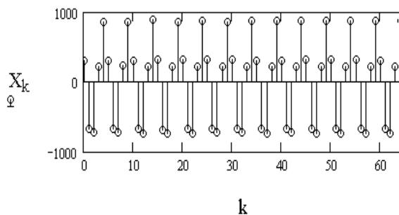
Рис. 3. Дискретные временные отсчеты принятого сигнала
