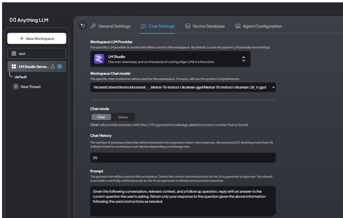
Рис. 17. Налаштування робочого простору AnythingLLM.
