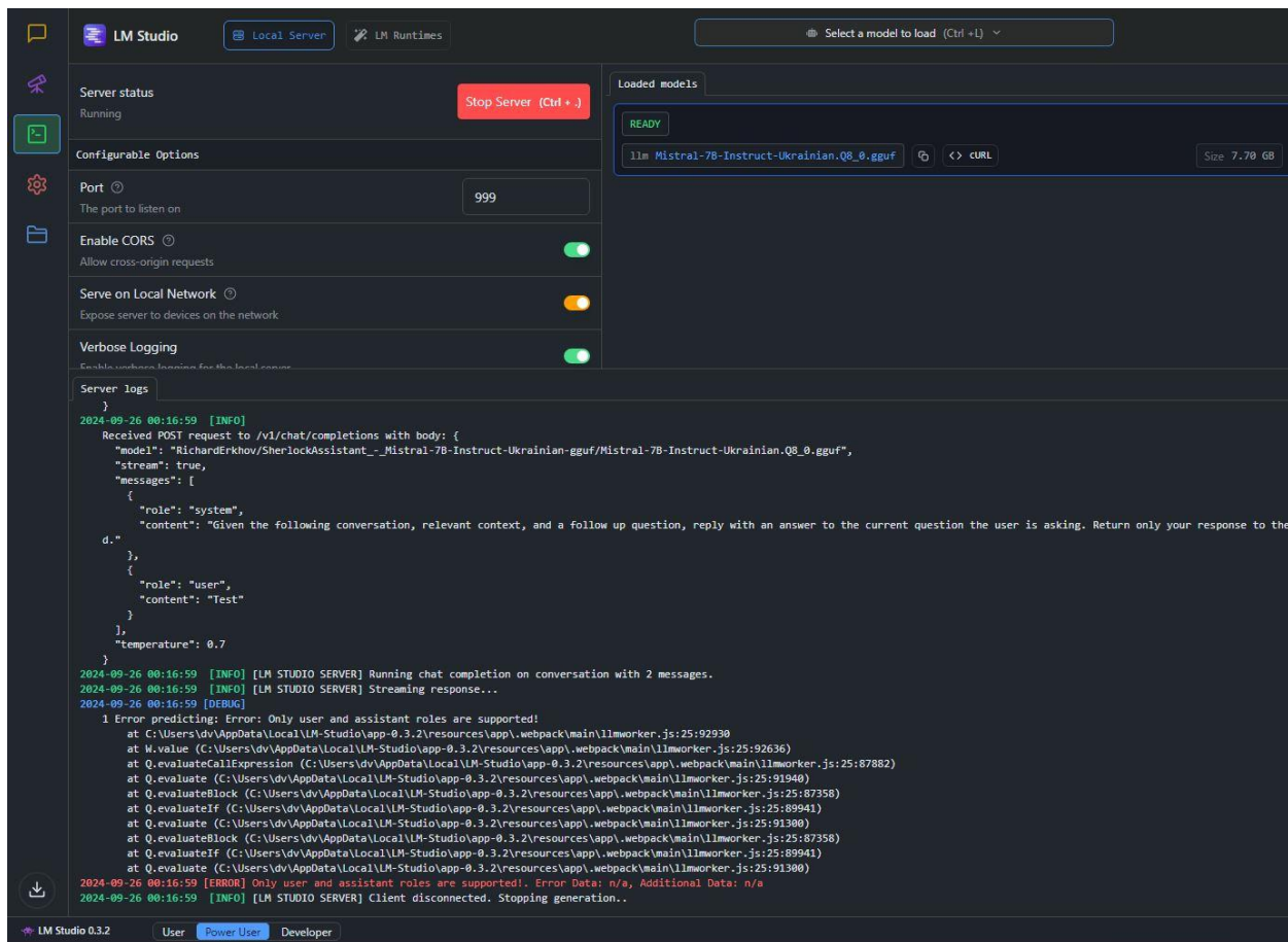
Рис. 19. Лог виконання запиту "Test"
