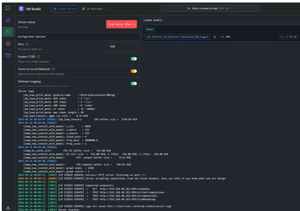
Рис. 14. Запуск функції Сервер на платформі LM Studio
