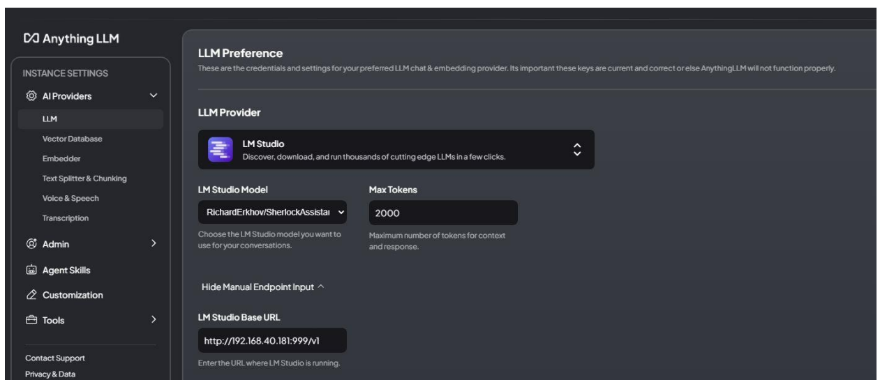
Рис. 16. Налаштування клієнтської частини AnythingLLM.
