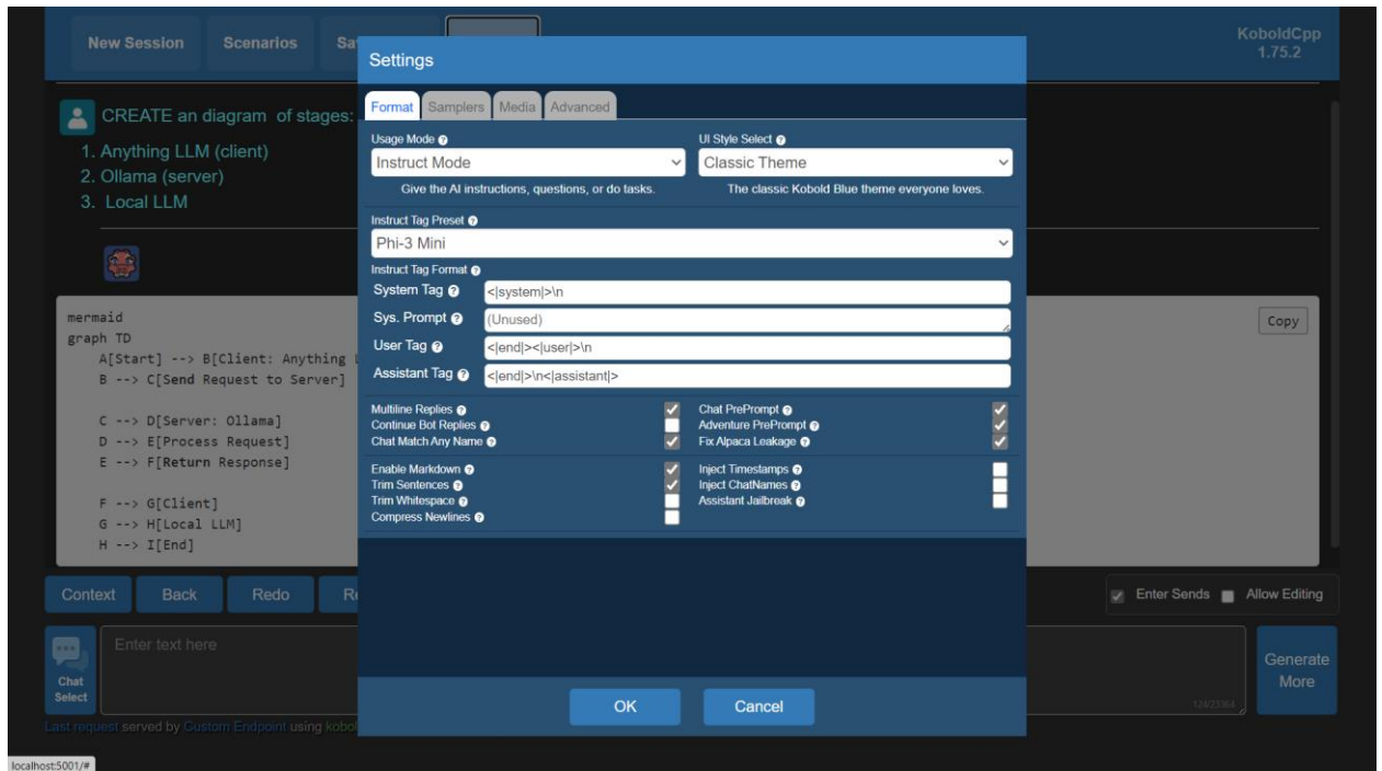
Рис. 10. Детальне налаштування фреймворку Koboldcpp за допомогою спеціальних параметрів у меню інтерфейсу “Settings”.
