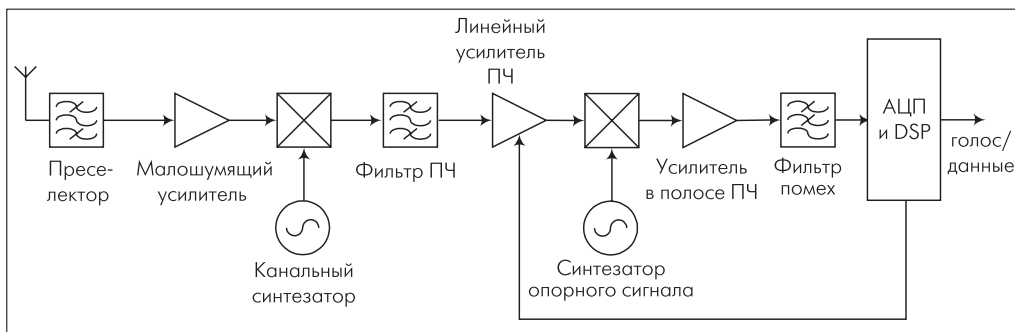
Рис. 5. Альтернативная схема цифрового приемника проекта SUNBEAM
