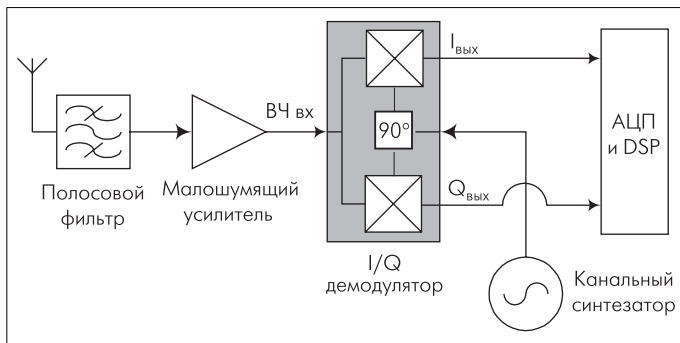
Рис. 6. Архитектура приемника прямого преобразования с ЦДО
